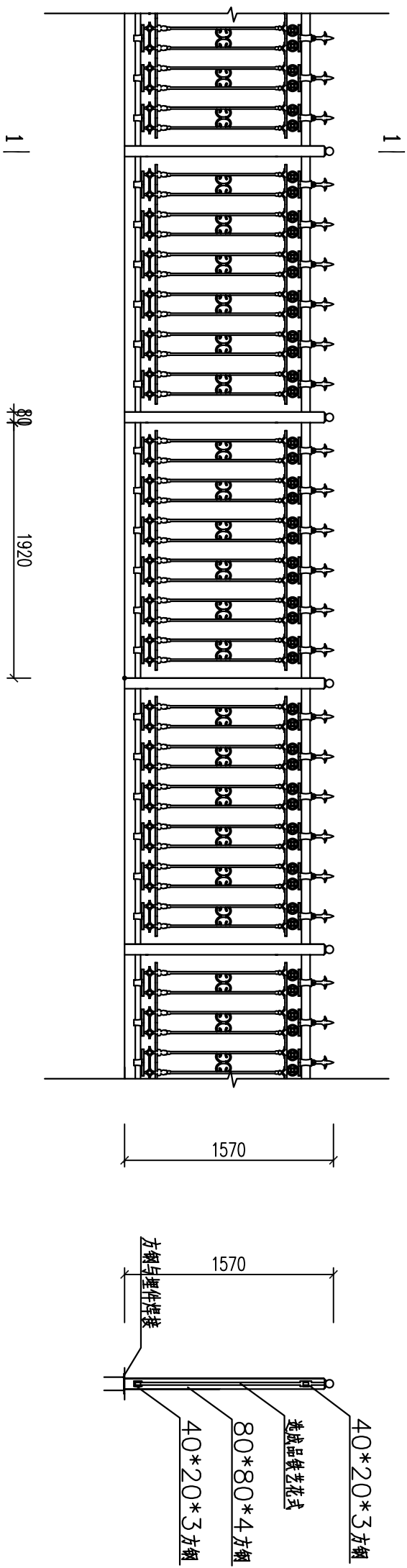
铁艺围墙立面图
