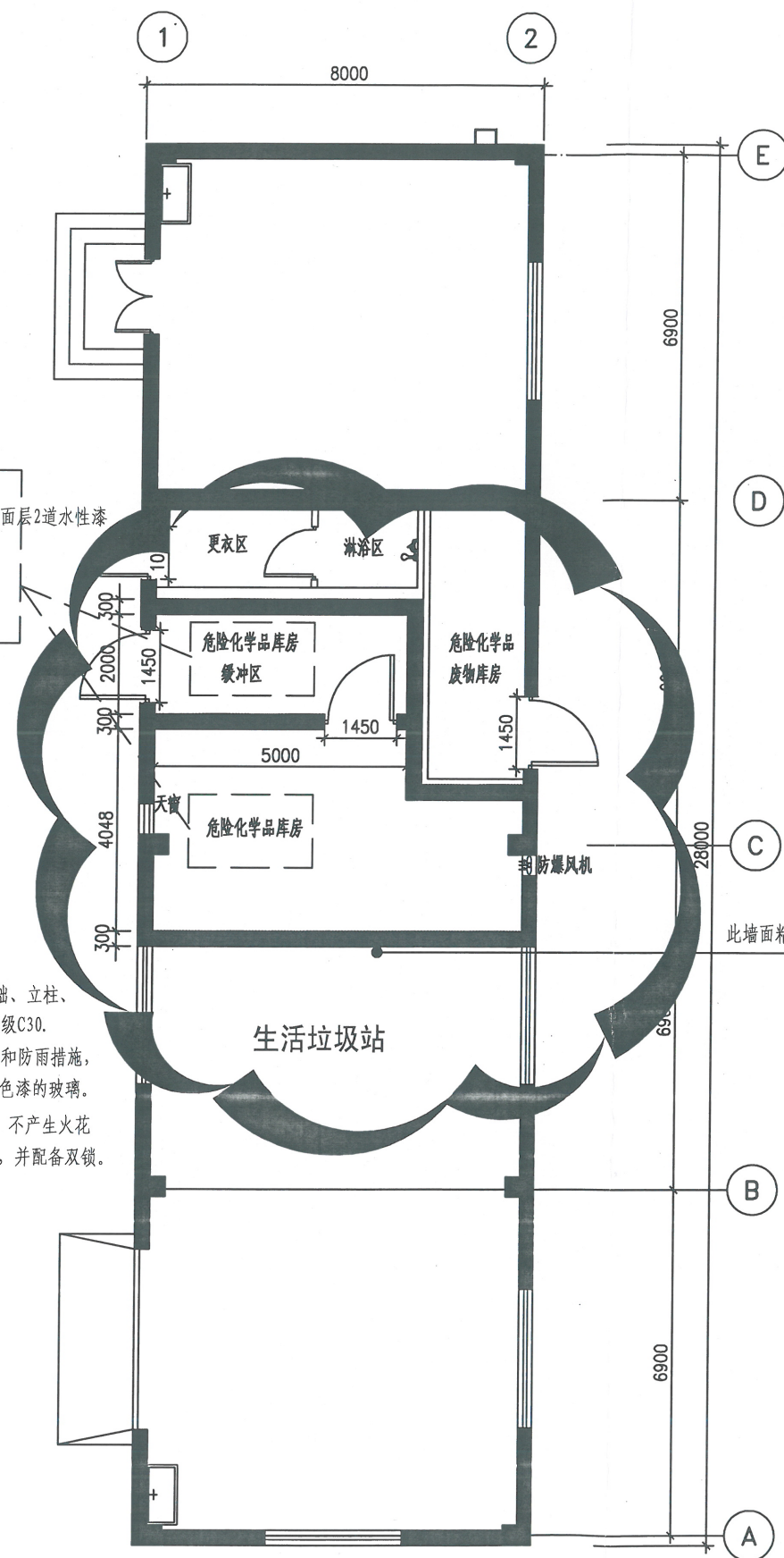
装饰平面图
