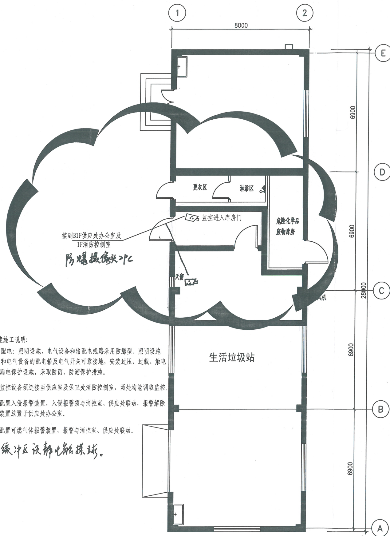
监控平面图
