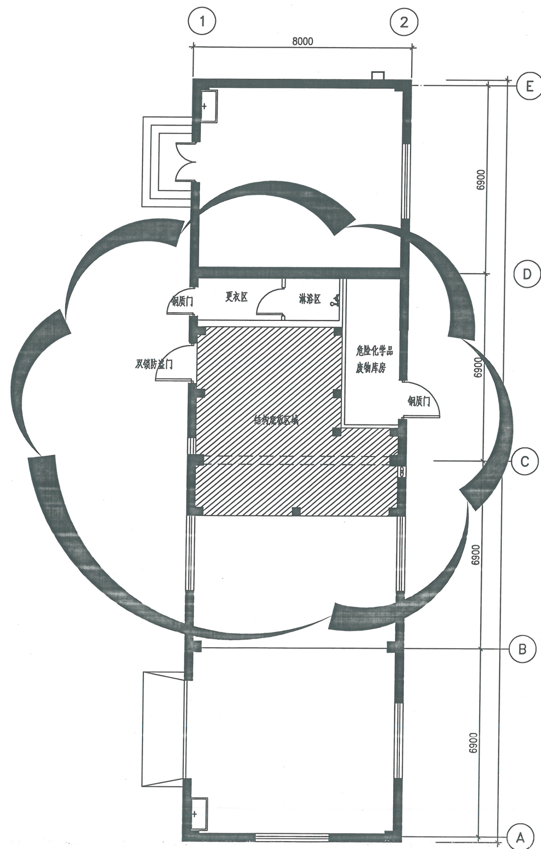
结构平面图
