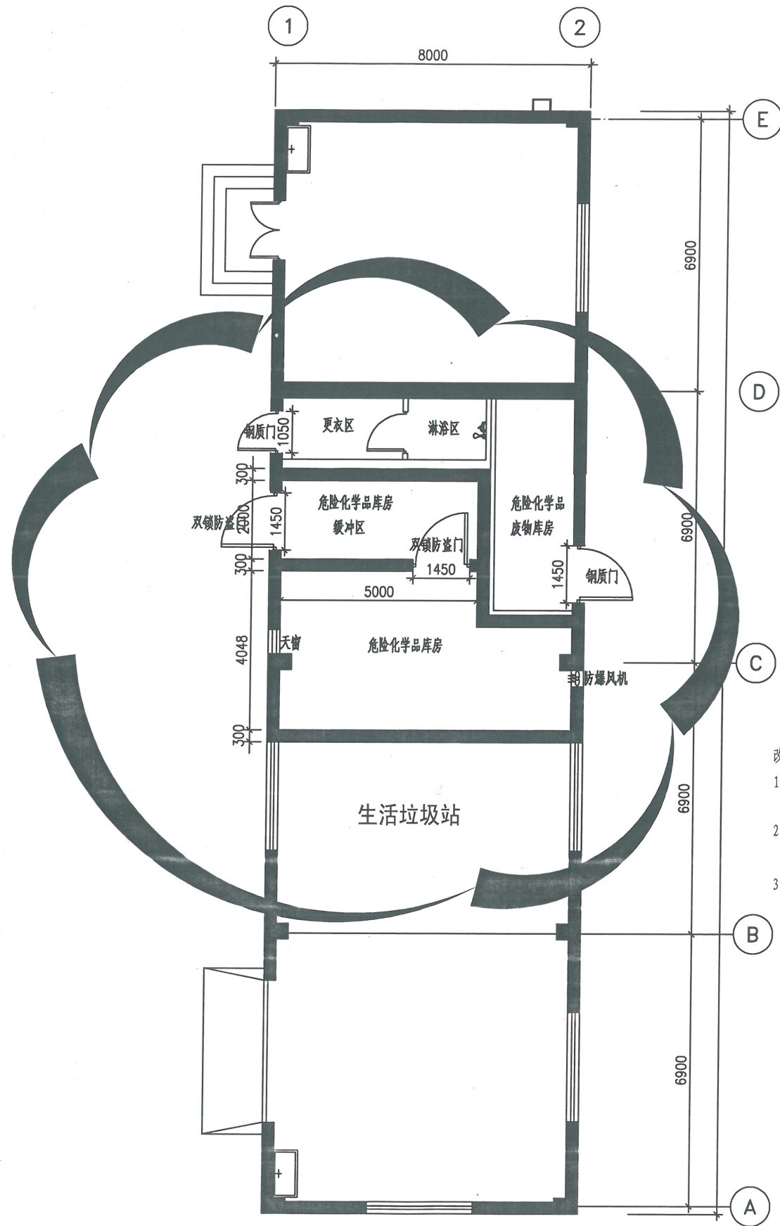
建筑平面图
