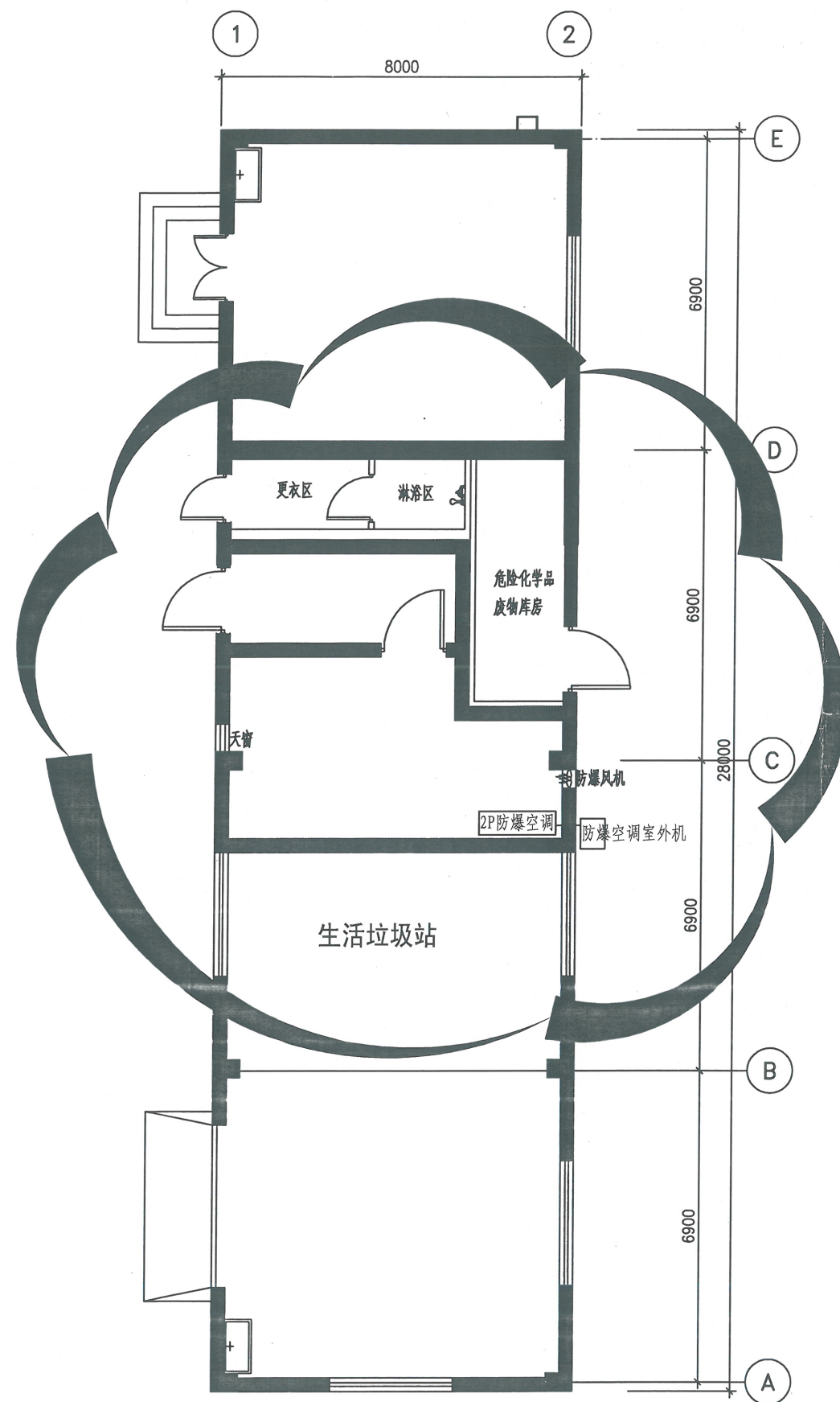
空调平面图
