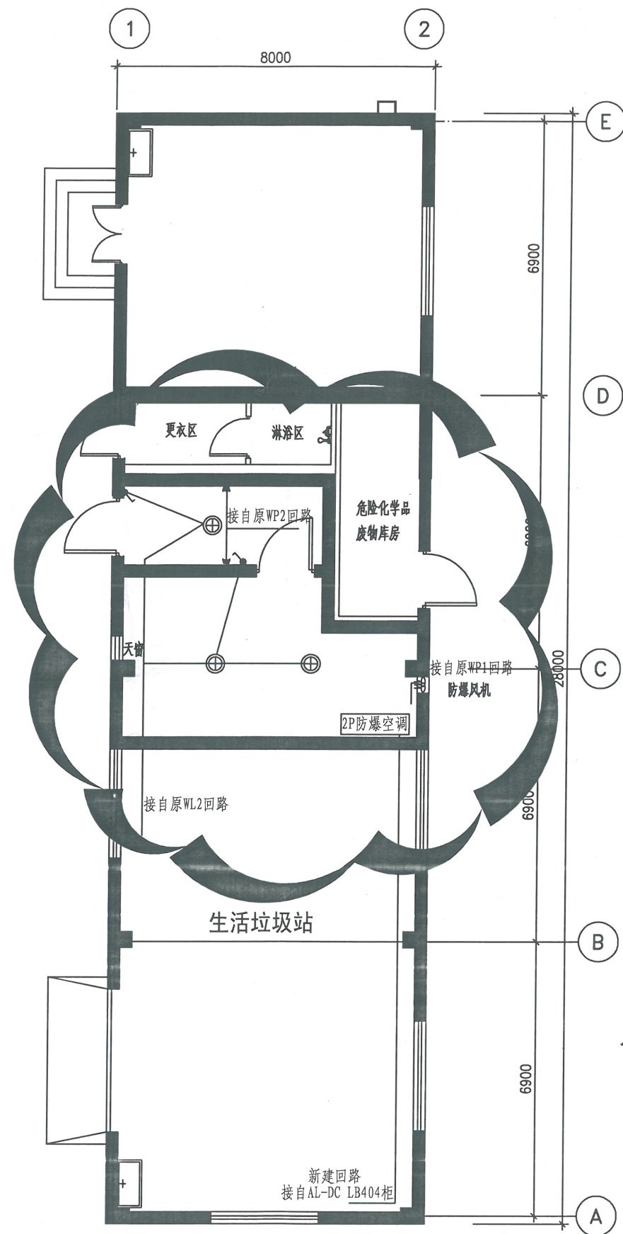
电气平面图
