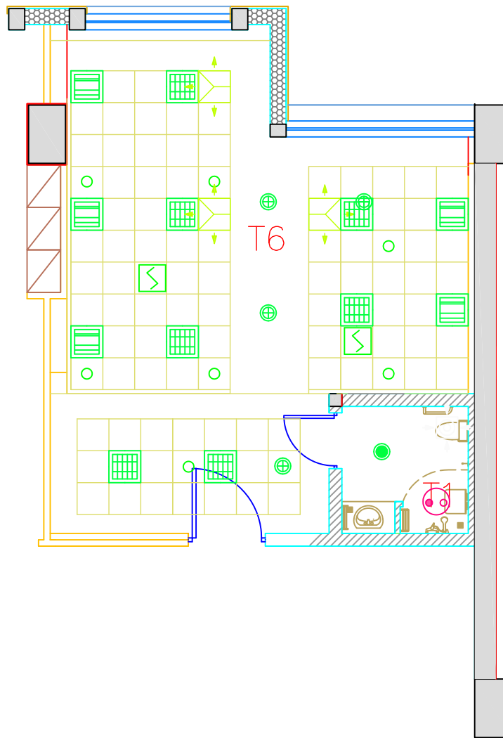
天花排布图
