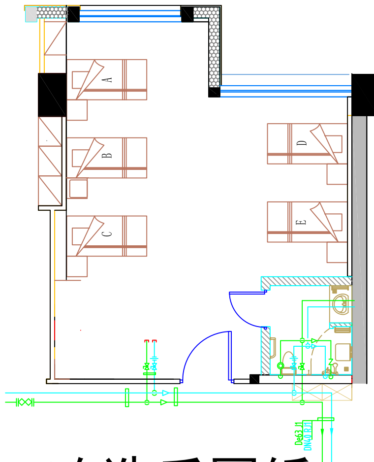
改造后图纸
