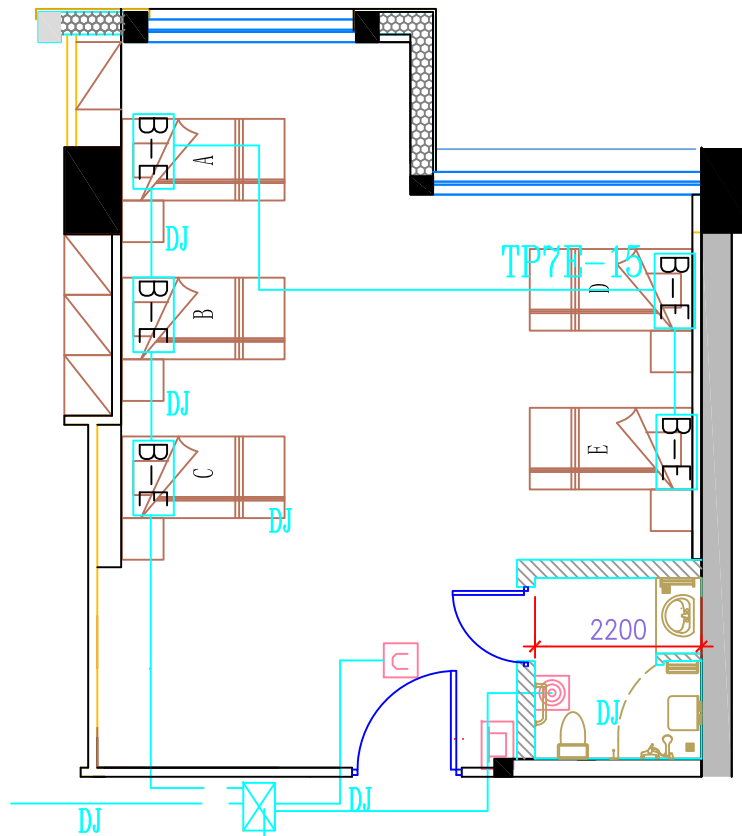
改造后图纸
