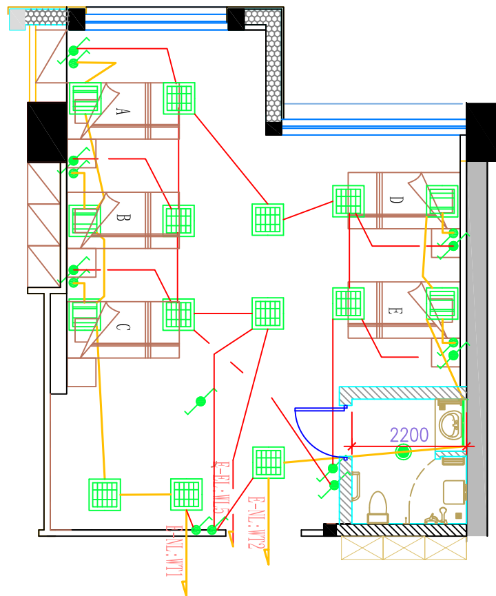
改造后图纸
