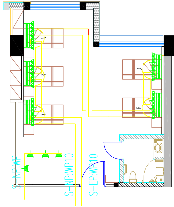
改造后图纸
