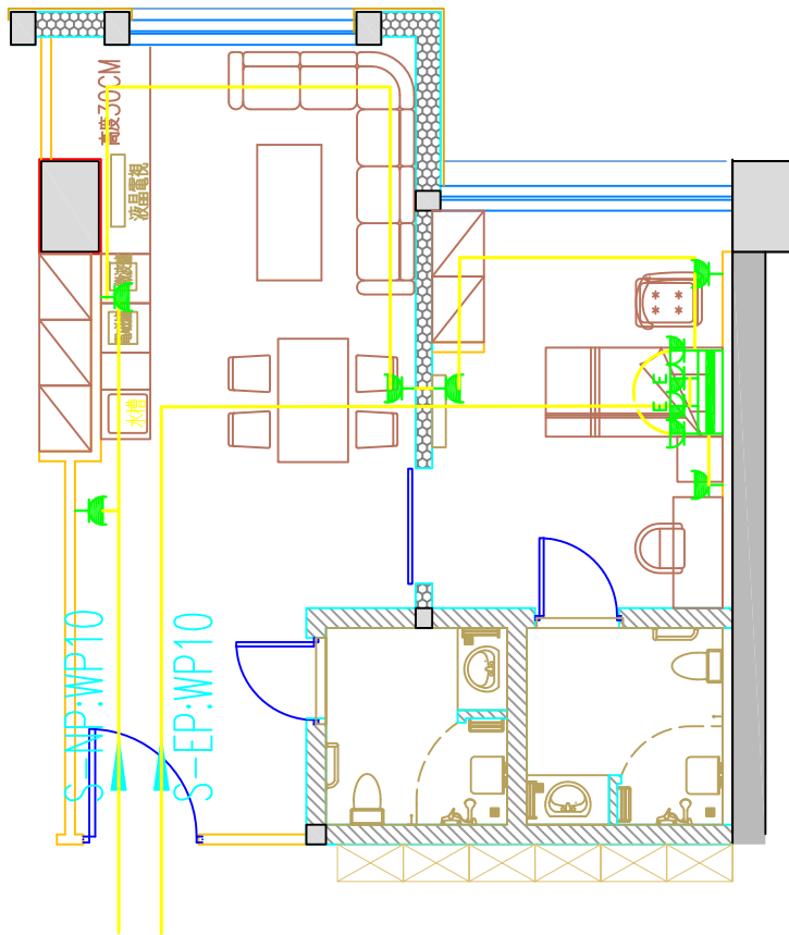
原平面图
