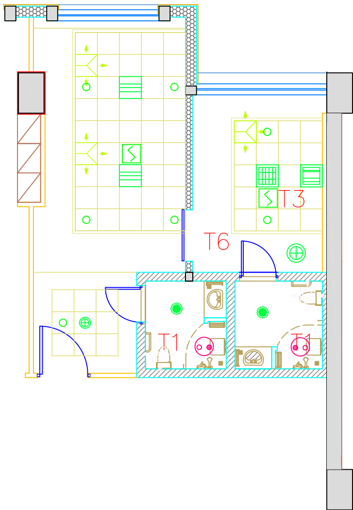
原平面图
