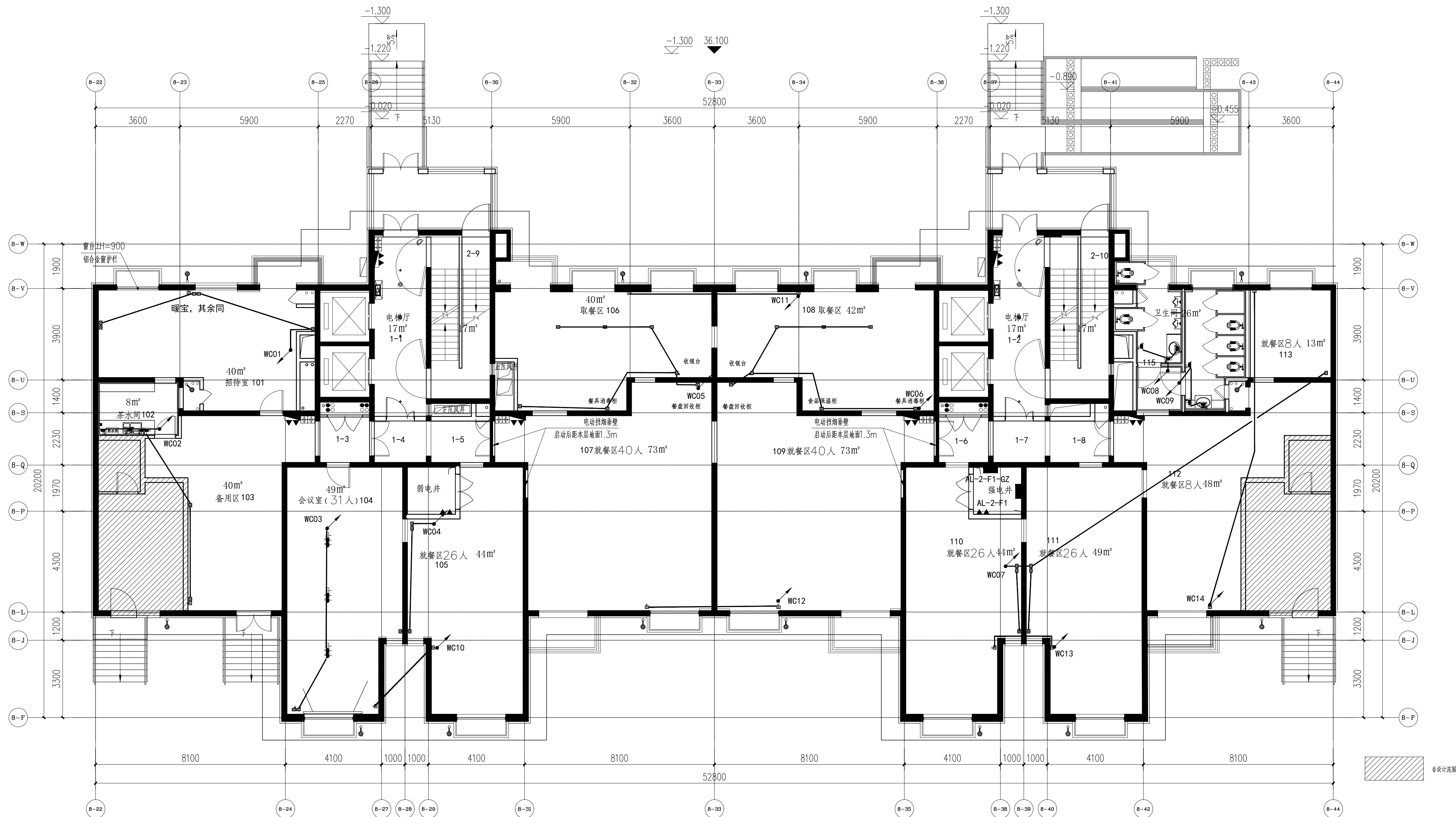
中塔首层普通插座连线图 1:100
